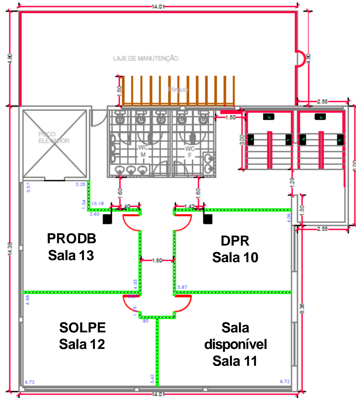
Planta 1º Pavimento área: 284,01 m 2
