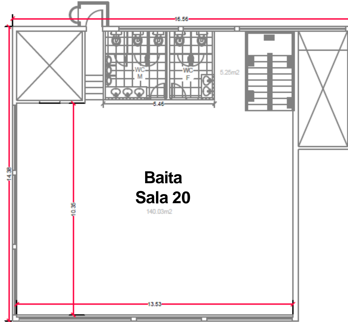
Planta Pavimento Cobertura
